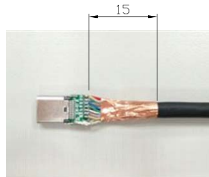
編織需跟雙面導電銅箔導通跟PCB板距離4~5mm
